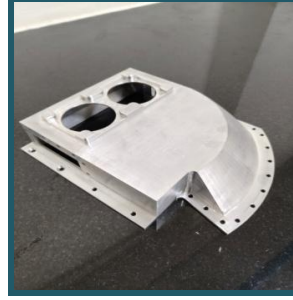
हीट एक्सचेंजर निकास प्लेनम
